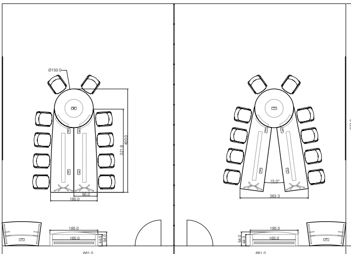
Länge 400 cm Breite 180 cm Öffnungswinkel 15°
